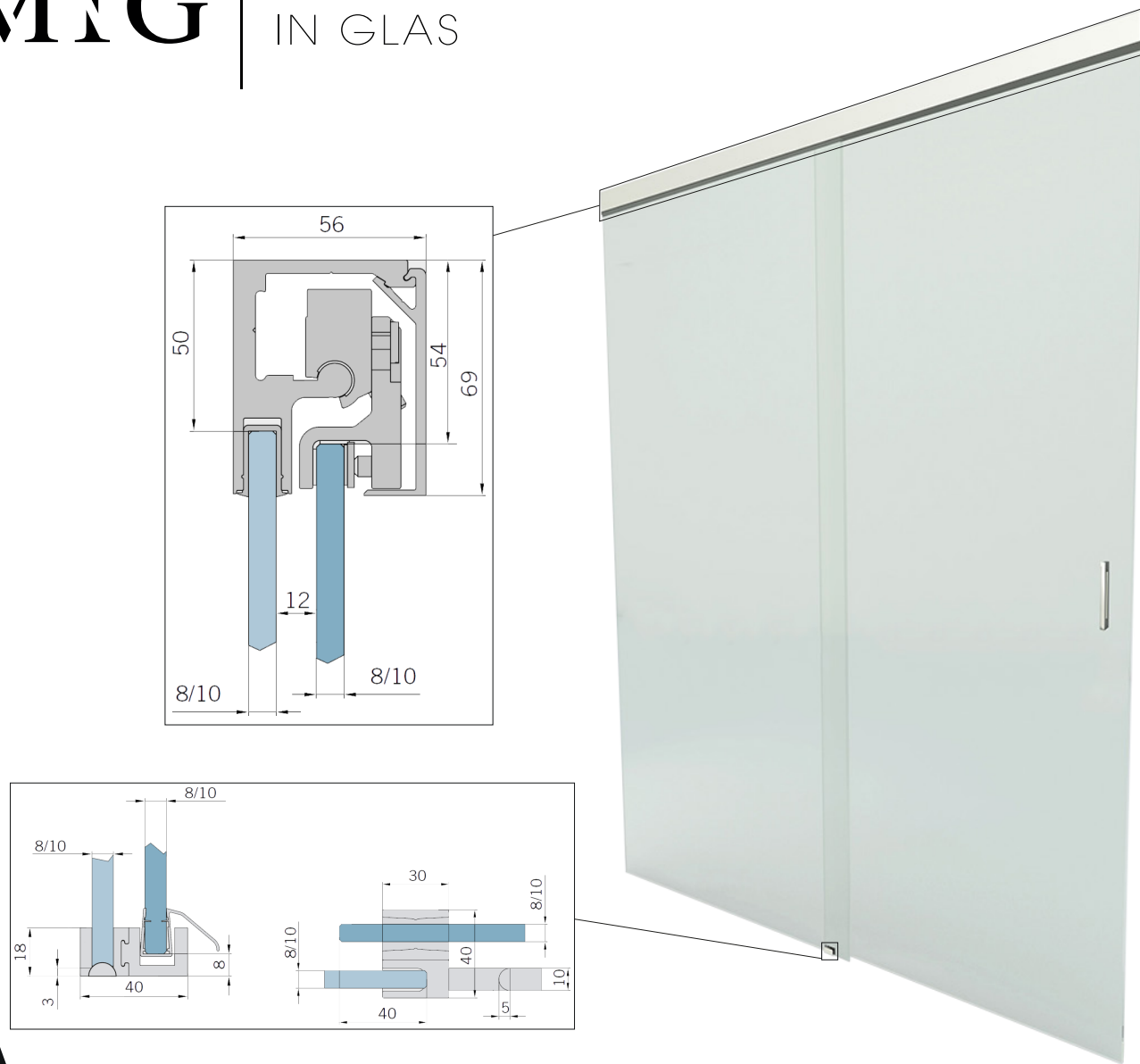
Glazen douche schuifdeur - premium
